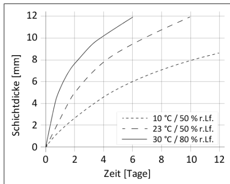
Diagramm 1: Durchhärtgeschwindigkeit Sikaflex®-268
