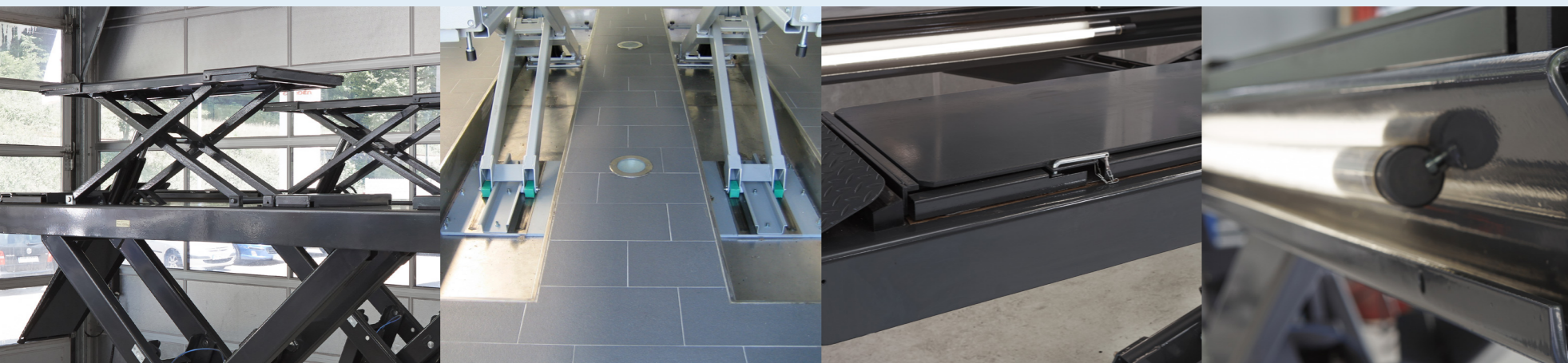
VERSIONE "PLUS AMS" (installazione a pavimento): con sollevatore integrato + pedane da assetto + traversa opzionale
