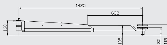
Long arm
