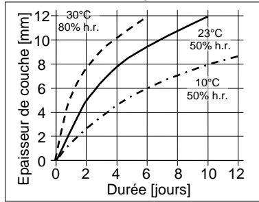
Diagramme 1: Vitesse de durcissement pour Sikaflex®-252
