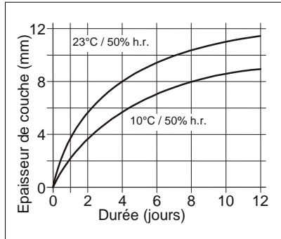
Diagramme 1: Vitesse de durcissement pour SikaTack® Drive
