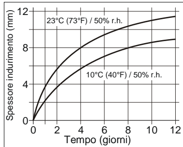
Diagramma 1: Velocità di indurimento di Sikaflex®-527 AT
