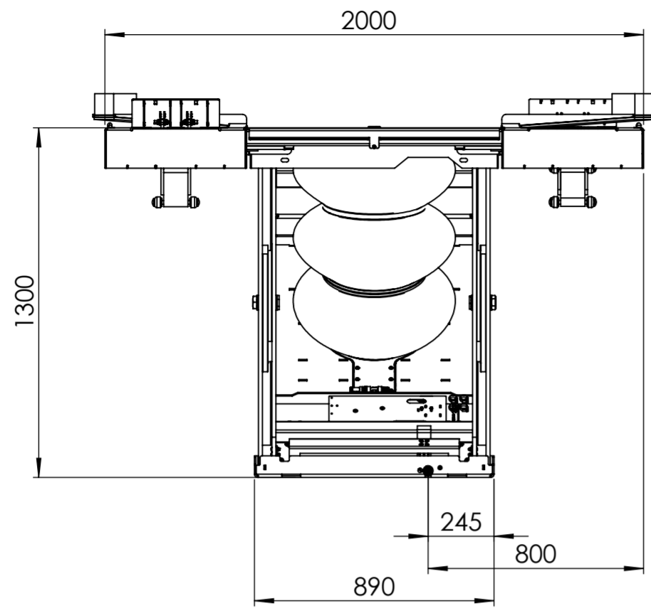
Bodenverschraubung/Bottom screwing
