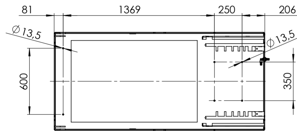
Bodenverschraubung/Bottom screwing
