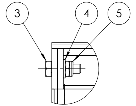
DETAIL A MAßSTAB 1 : 2
