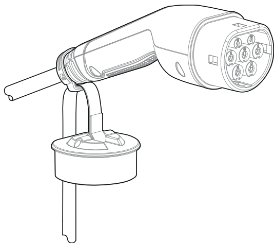
Presa del veicolo di tipo 2 con tappo e cinghia
